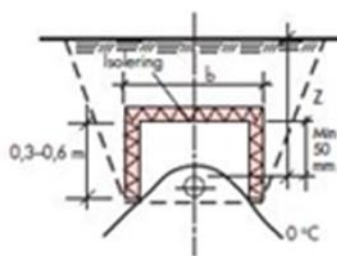
Hästskeformad isolering.
