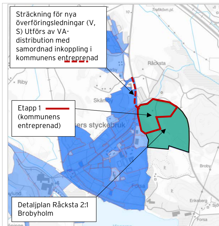
Figur 1. Investeringsbeslutet avser exploatering av den första utbyggnadsetappen i detaljplanen Räcksta 2:1 Brobyholm inklusive nya överföringsledningar för vatten- och spillvatten. Röd markering redovisar den första utbyggnadsetappen.
